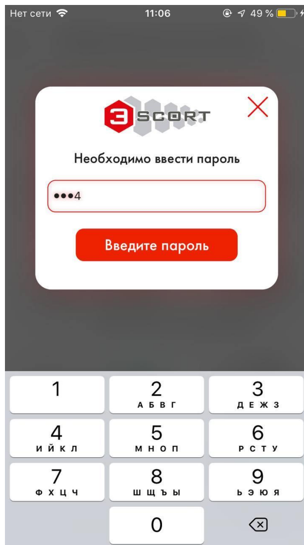
Рис. 12 Ввод пароля
