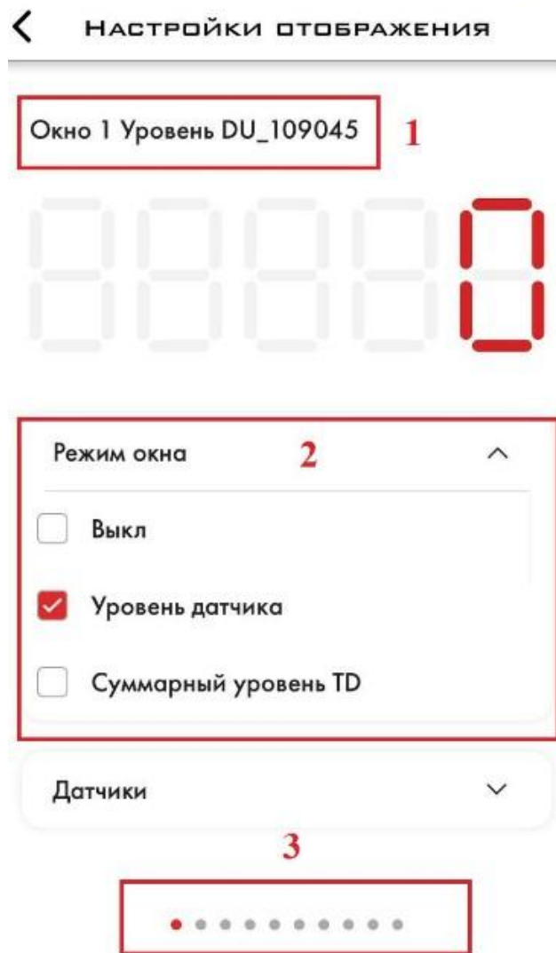
Рис. 57 Настройки отображения
