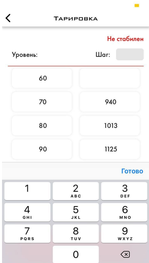
Рис. 51 редактирование ячеек
