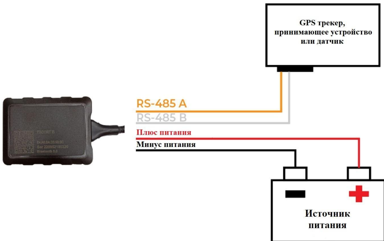
Рис. 9 Схема подключения И-5
