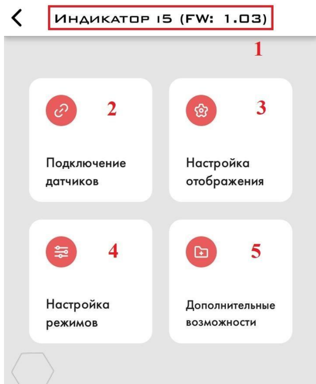
Рис 66 Подключение датчиков 2
