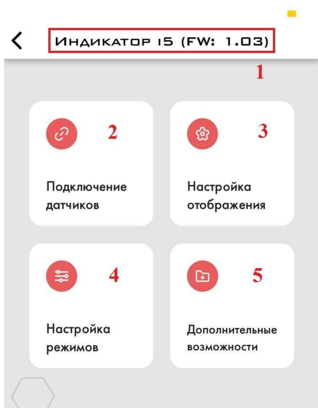
Рис. 40 Настройка режимов (4)
